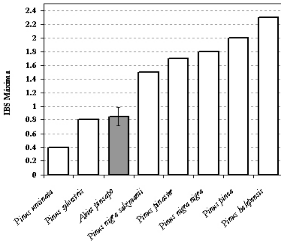
Figuras 2A y 2B. Ejemplo de diagrama bioclimático de Montero Burgos y González Rebollar para la
