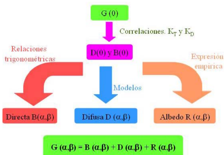
Figura 1. Esquema para el cálculo de la irradiancia.
